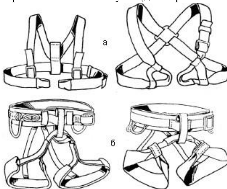
Рис. 1. Індивідуальні страхувальні системи різної конструкції
