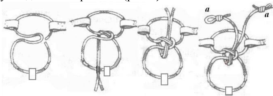
Рис.4. Блокування страховальної системи вузлом подвійний булінь; а - «вуси» для самострахування
