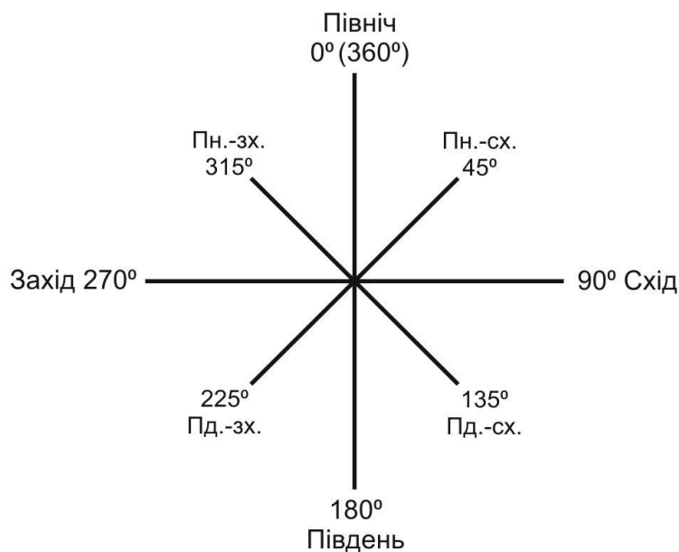
Рис.1. Роза вітрів
