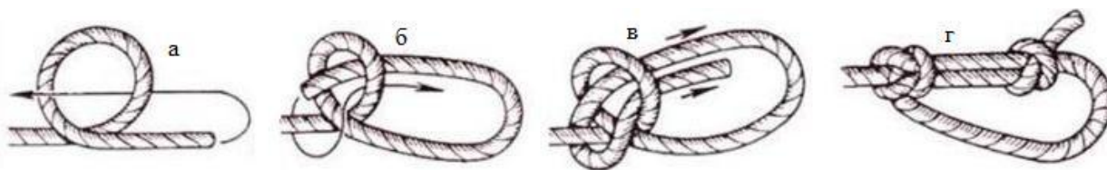
Рис. 9. Вузол «булінь»: а-в – етапи в'язання вузла, г – вузол «булінь» з контрольним вузлом
